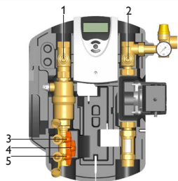
Exemple: Station solaire avec unité de vidange et de remplissage
