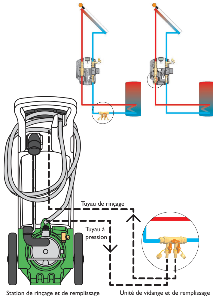
Station de rinçage et de remplissage
