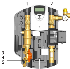
Ejemplo: estación solar con la unidad de válvula llenado y vaciado
