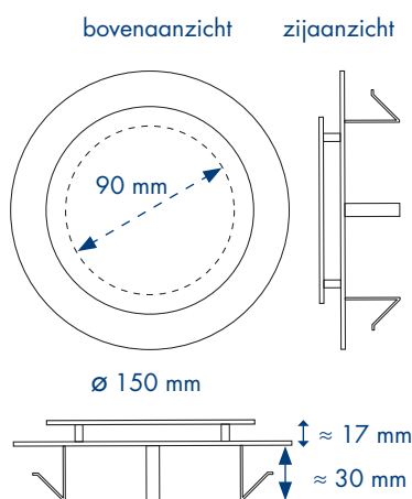
rond met klem-bevestiging
