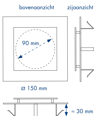
4-kant met klem-bevestiging
