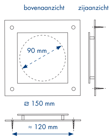
4-kant met schroef-bevestiging
