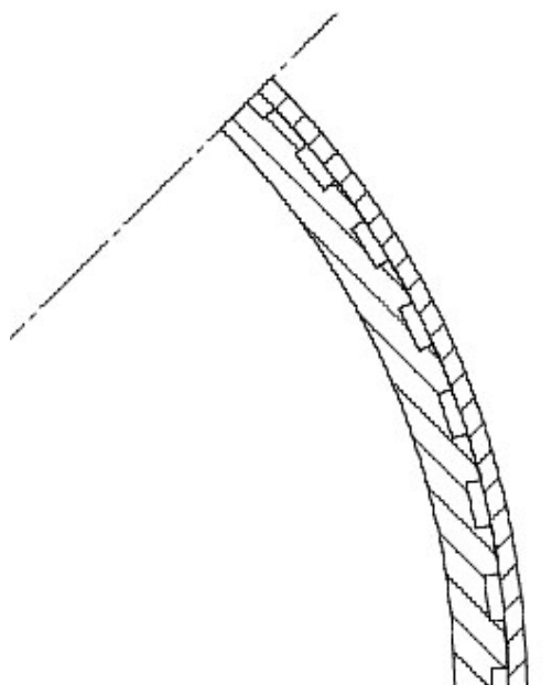
Doorsnede douche WTW met lekdetectiekanaaltjes
