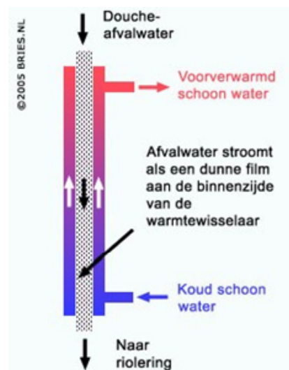
Werking douche-WTW
