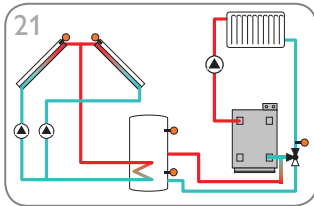
Systeem voor verwarming met zonne-energie met oost-/westdak en verhoging van de teruglooptemperatuur van de verwarmingskring (pagina 51)
