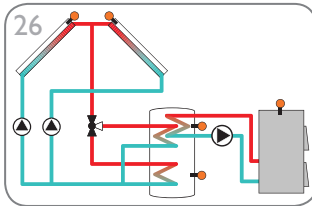
Systeem met oost-/westdak, reservoir met stratificatie en bijverwarming via ketel met vaste brandstof (pagina 65)
