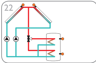
Systeem voor verwarming met zonne-energie met reservoir met stratificatie en oost-/westdak (pagina 53)
