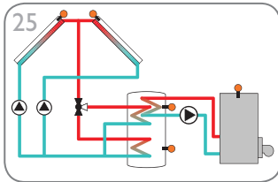
Systeem met oost-/westdak, reservoir met stratificatie en thermostatische bijverwarming (pagina 62)
