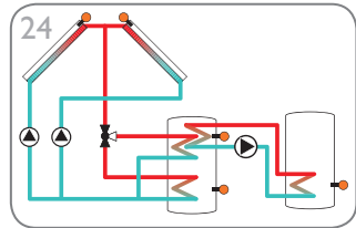
Systeem voor verwarming met zonne-energie met oost-/westdak, reservoir met stratificatie en uitwisseling van warmte (pagina 59)
