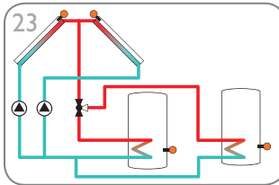
Systeem voor verwarming met zonne-energie met oost-/westdak en 2 reservoirs (ventiellogica) (pagina 56)
