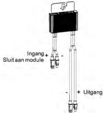
Afbeelding 1: Connectoren van de power optimizer
