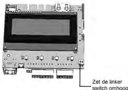
Afbeelding 21: RS485-afsluitschakelaar
