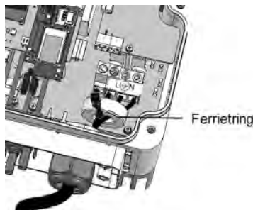
Afbeelding 8: AC-aansluiting
