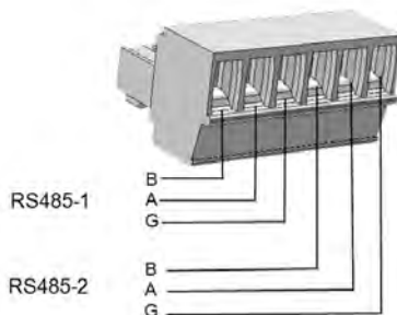
Afbeelding 19: RS485-klemmenblok
