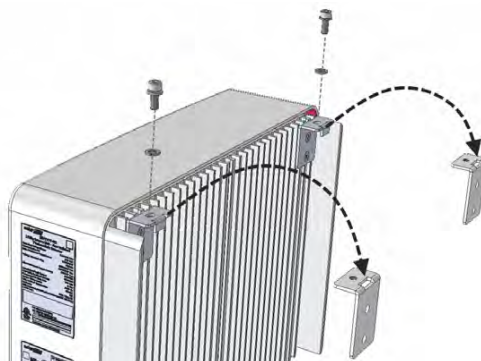
Afbeelding 24: Montagebeugels
