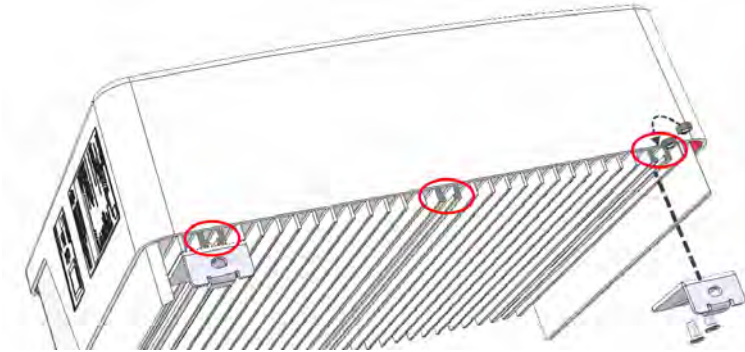
Afbeelding 5: De beugels van de omvormer monteren
