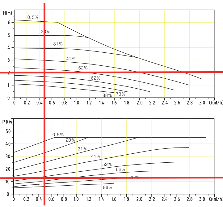
CPA-E55/xx-xxx S PWM signaal
