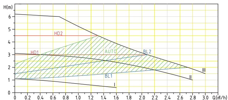
Circulateur CPA-E55/xx-xxx
