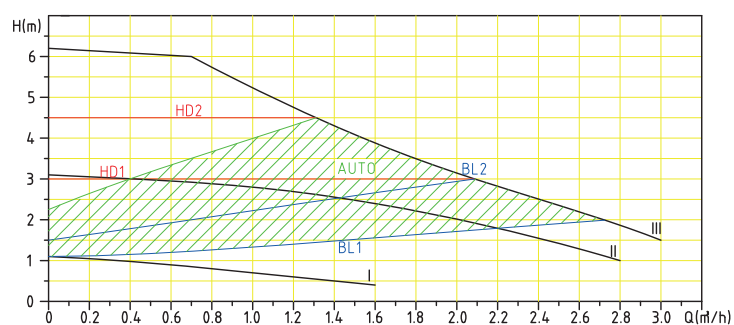
CPA-E55/xx-xxx circulatiepomp
