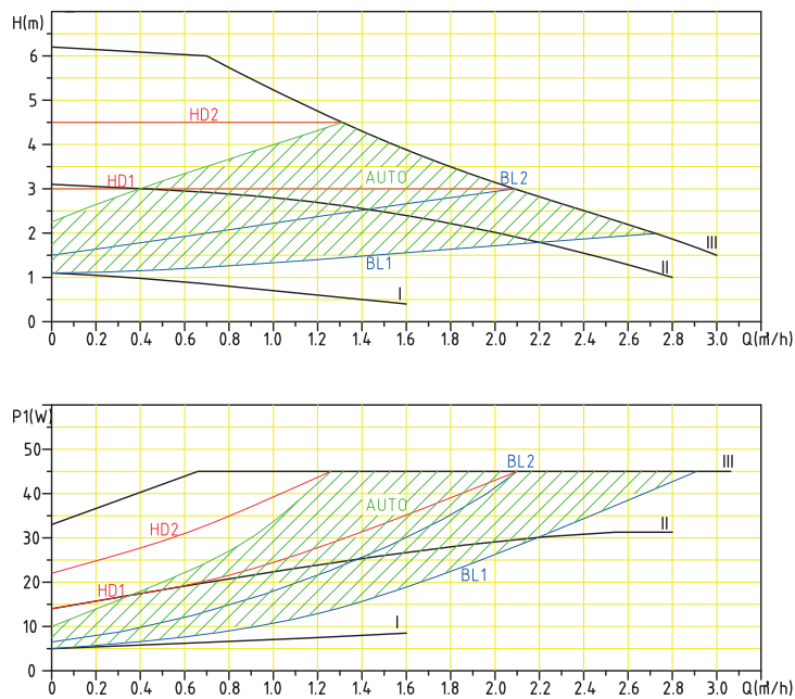
CPA-E55/× ×-xxx Umwälzpumpe
