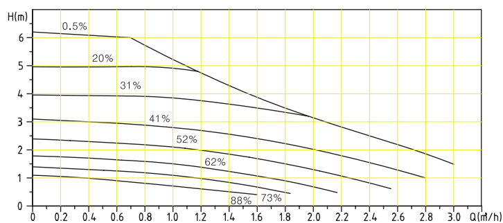
CPA-E55/xx-xxx S PWM signaal
