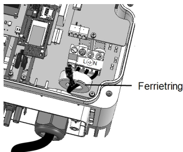
Afbeelding 23: AC-aansluitingen
