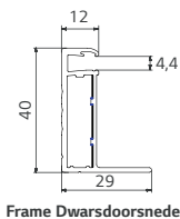
Frame Dwarsdoorsnede
