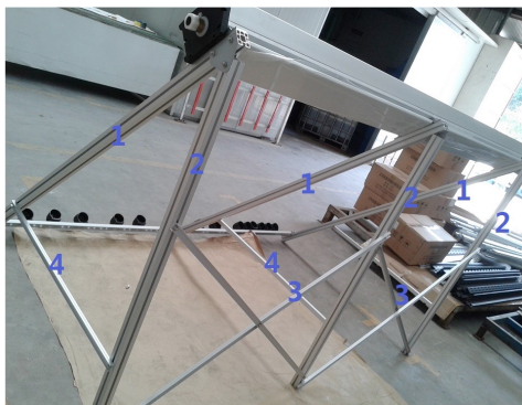
2. Alle onderdelen na de montage van de platdak frame.
